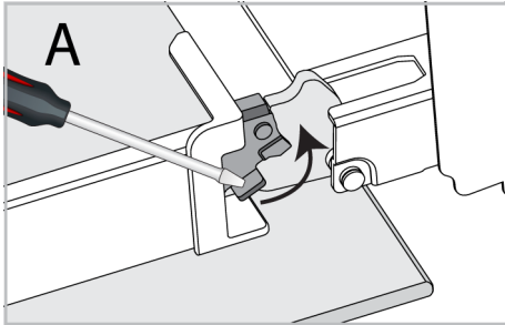
İllüstrasyon 1: Menteşe kilidi - kapalı pozisyon
