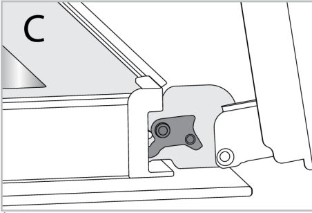
İllüstrasyon 6: Menteşe kilidi - açık pozisyon
